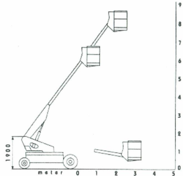
Vlucht diagram AFRON hoogwerker R.S.T. 3
